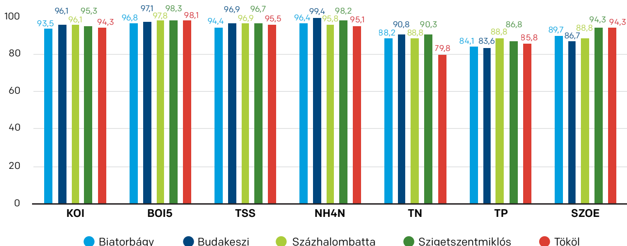
Átlagos szennyezőanyag eltávolítási hatékonyság az agglomerációs szennyvíztisztító telepeken (%)
