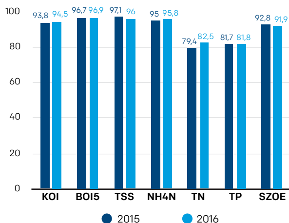
Átlagos szennyezőanyag eltávolítási hatékonyság (%) BKSZTT
