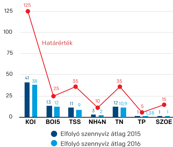
BKSZTT elfolyó szennyvíz minőség (mg/l)
