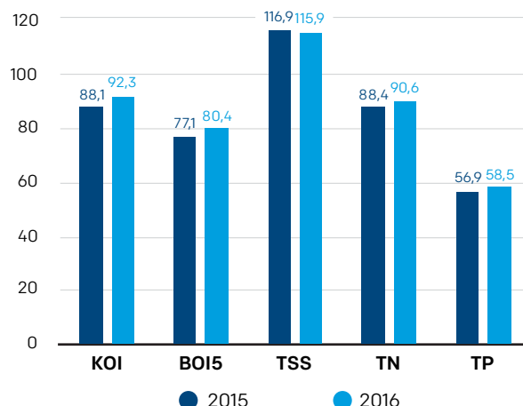
Befolyó szennyvíz kapacitás kihasználtsági arány (%) BKSZTT
